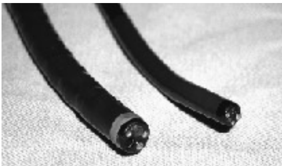
左：通常の胃カメラ 外径 9.0 右：経鼻用胃カメラ 外径 5.9
